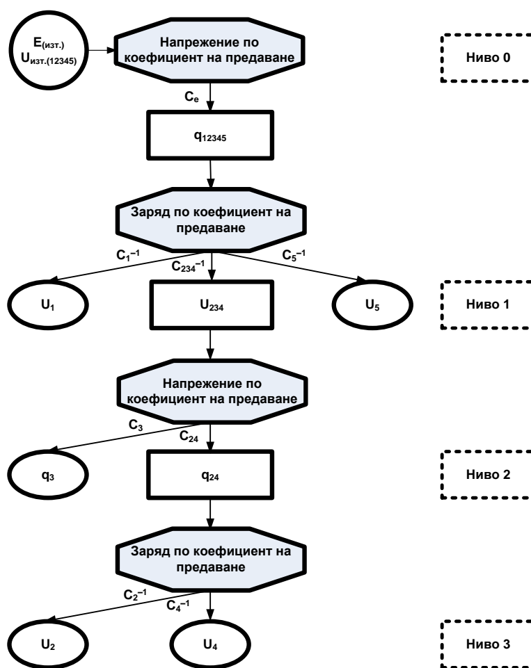
Фиг. 4. Еквивалентна дървовидна структура на смесено съединени кондензатори за определяне на зарядите и напреженията (в обратна посока - надолу).
