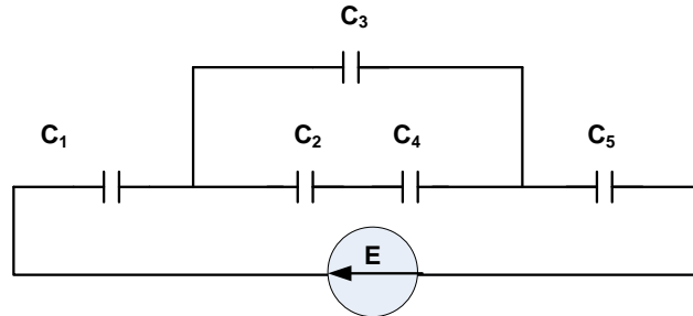
Фиг. 1. Схема на електростатична верига със смесено съединени кондензатори.
