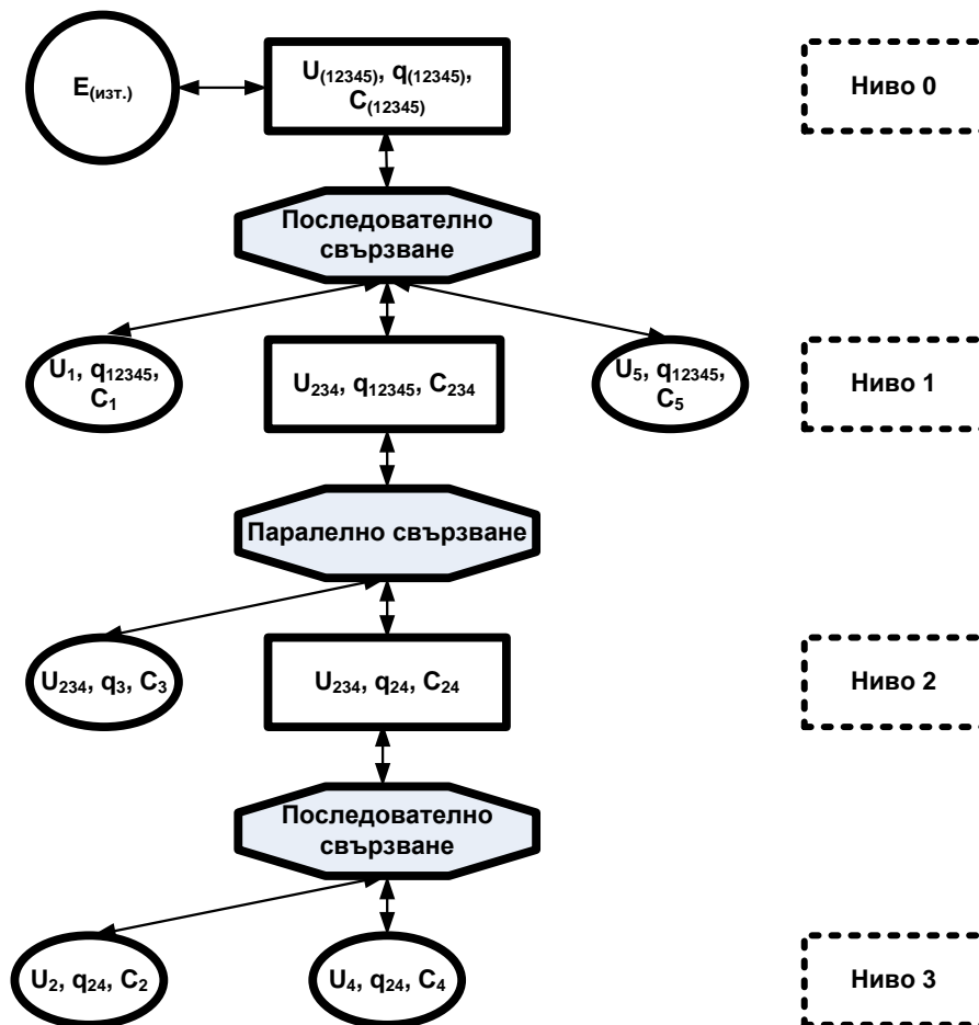
Фиг. 2. Дървовидна схема на смесено съединени кондензатори.
